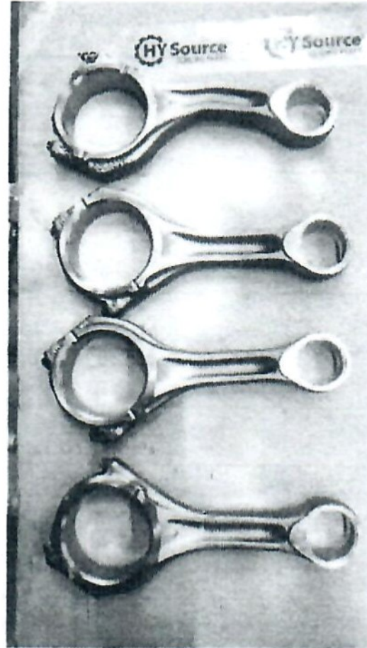
Biela do 4º cilindro sofreu empenamento pelo calço hidráulico
