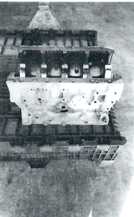
Foto geral bloco do motor.
