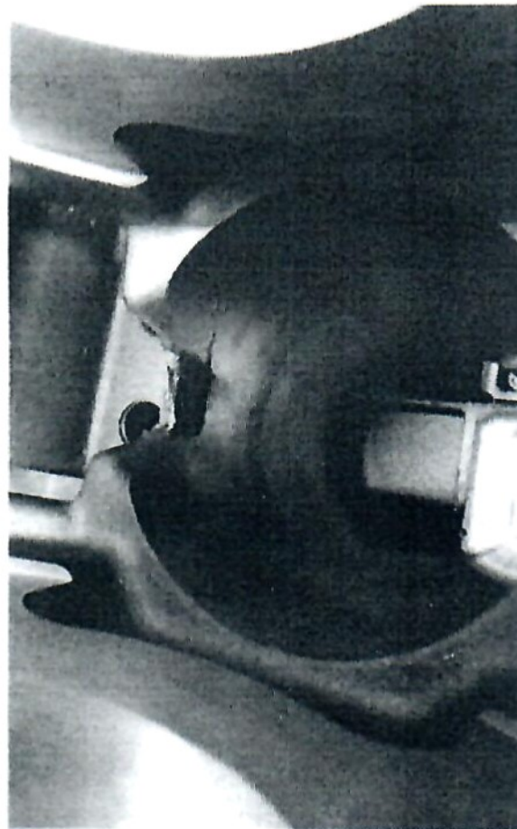
Fratura frágil na parte inferior do cilindro.
