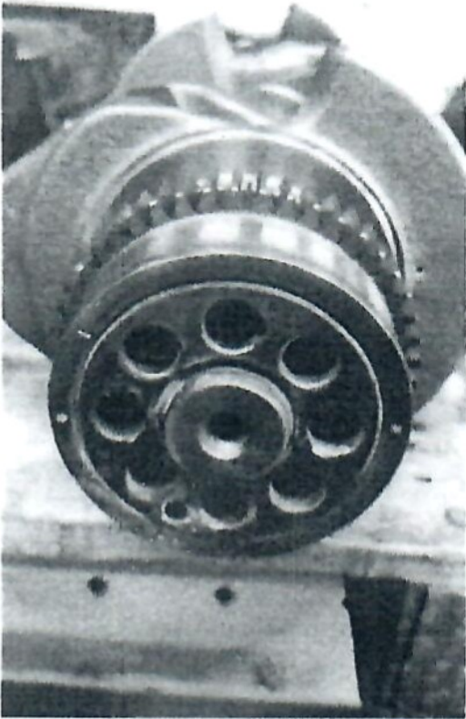
Virabrequim danificado por quebra dos parafusos
